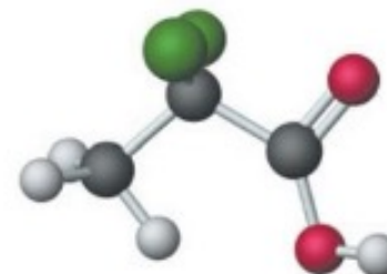
CH 3 Cl 2 COOH Acide 2,2-dichloropropanoïque
